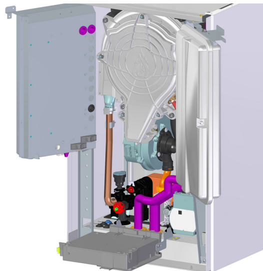
fig. 62 - accesso ai componenti interni
