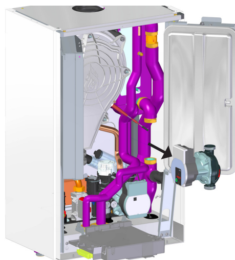
fig. 65 - Sostituzione/manutenzione circolatore della pompa di calore
