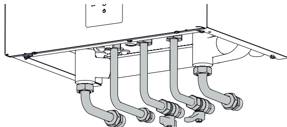
fig. 4 - Kit idraulico montato
